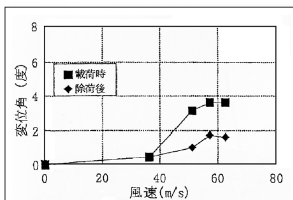
図 1：風速とポールの変位角度の関係 （載荷試験から算出）
