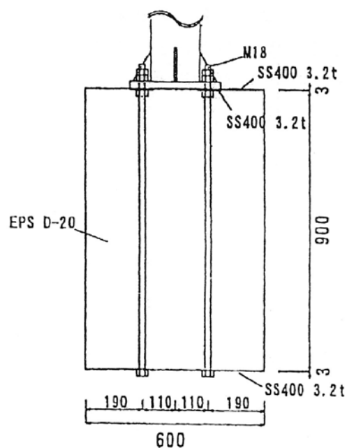
図.サットワンベースタイプのボルト設置後の概要図
