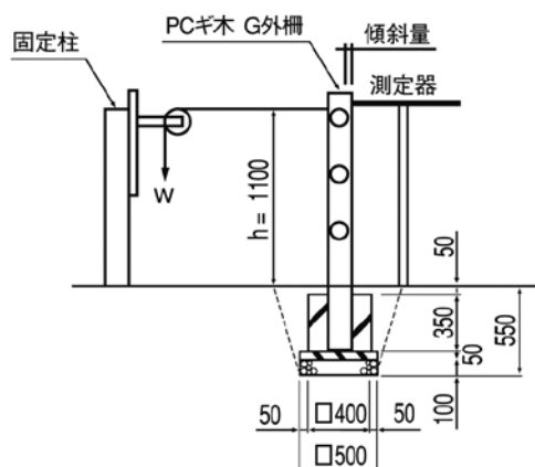
2.3.1 G外柵試験図
